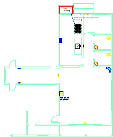
Planta PPCI Escala: 1/50
