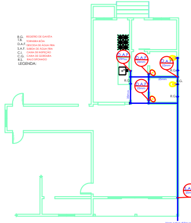
Planta Hidráulica Escala: 1/50
