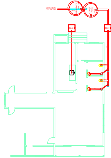
Planta Sanitário Escala: 1/50
